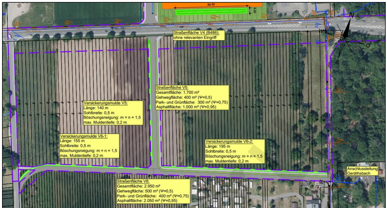
Abbildung 25: Planung Entwässerung, Verkehrsflächen V5 und V6 (Plan-Nr. W 1.3)
