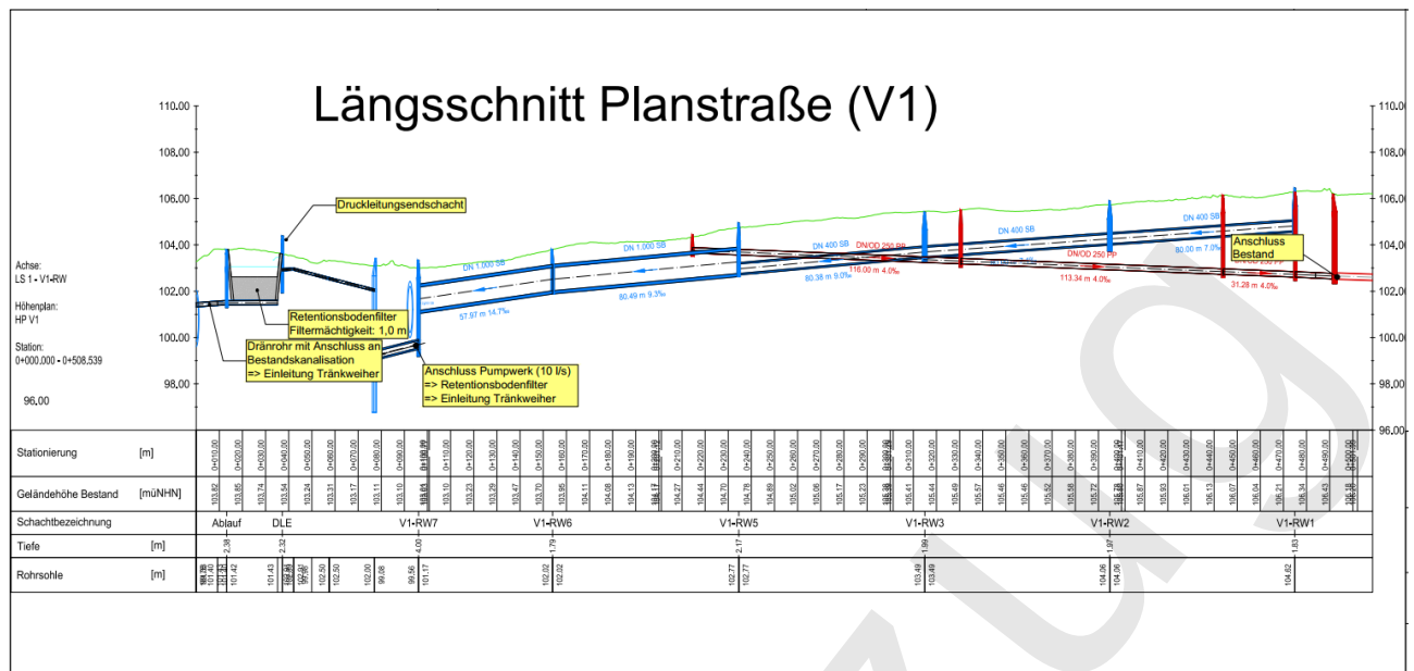
Abbildung 22: Längsschnitt Erschließungsstraße V1 ( Plan-Nr. W 2.1 )
