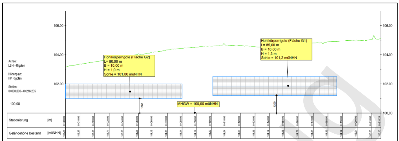
Abbildung 17: Längsschnitt der Rigolen ( Plan-Nr. W 2.4 )
