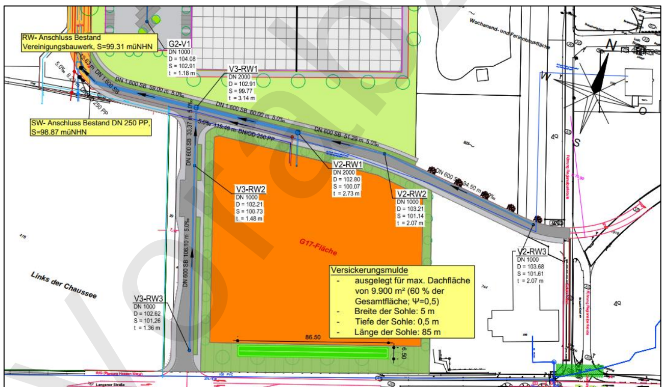
Abbildung 23: Entwässerungsplan Verkehrsflächen V2, V3 und Gewerbefläche G17 (Plan-Nr. W 1.2 LP)
