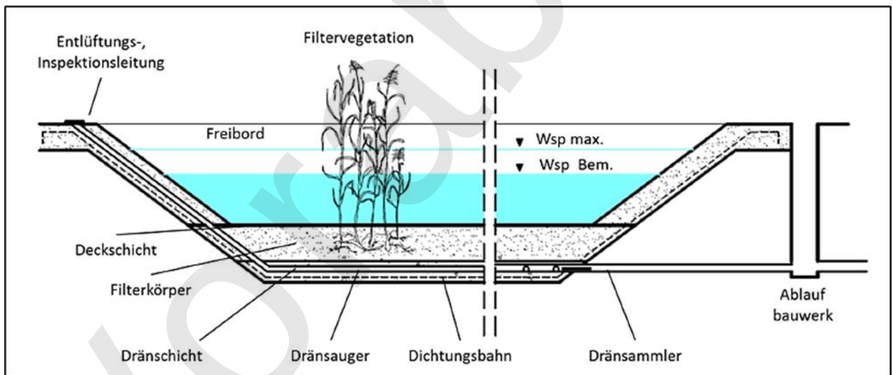
Abbildung 24: Retentionsbodenfilterbecken Querschnitt (/U30/)
