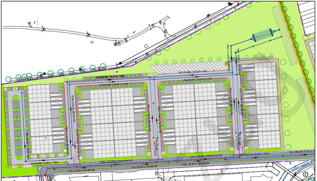
Abbildung 19: Fläche G1 – Kanalnetz (Plan-Nr. W 1.2)
